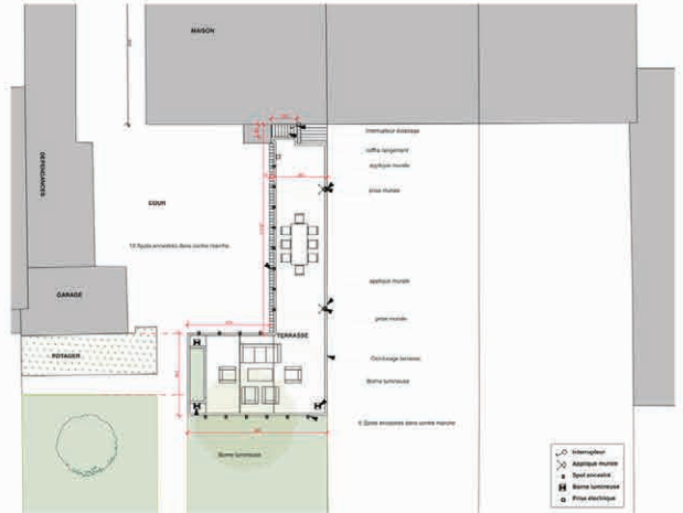
PLAN PROJET - AMÉNAGEMENT EXTÉRIEUR
